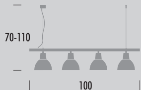
LORA Z4 B Chandelier 112-00..-001470 4xE27
