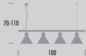
LINA Z4 B Chandelier 112-00...-001480 4xE27
